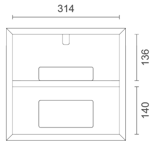
Voorkant (binnen)
