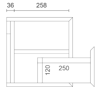
Zijkant (binnen)
