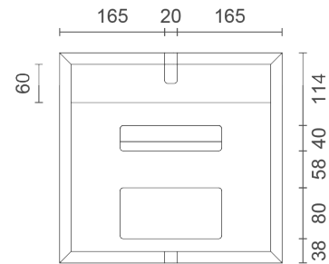
Achterkant
